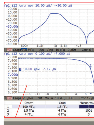
Развертка с линейным изменением мощности на одной частоте
